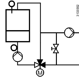
Поддерживаемая обратка бойлера при помощи смешивательного клапана
