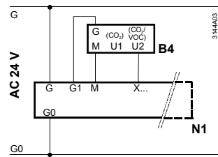
Схема 3 и 4: Измерение CO 2 /VOC- и CO 2
