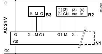
Схема 3 и 4: Измерение CO 2 /VOC- и CO 2
