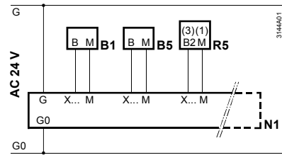
Схема 1: Подключение пассивных источников сигналов
